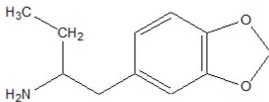
3,4-(Methylenedioxyphenyl)-2-butanamine BDB
